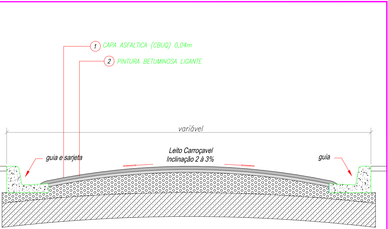
PERFIL TRANSVERSAL DA RUA
