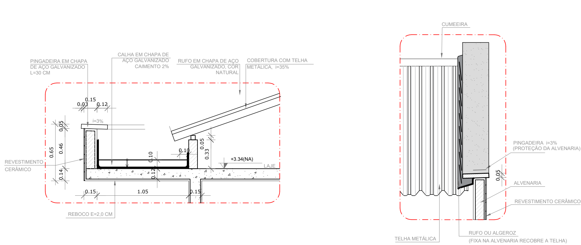
1 DETALHE 1 - CALHA ESCALA 1/25
