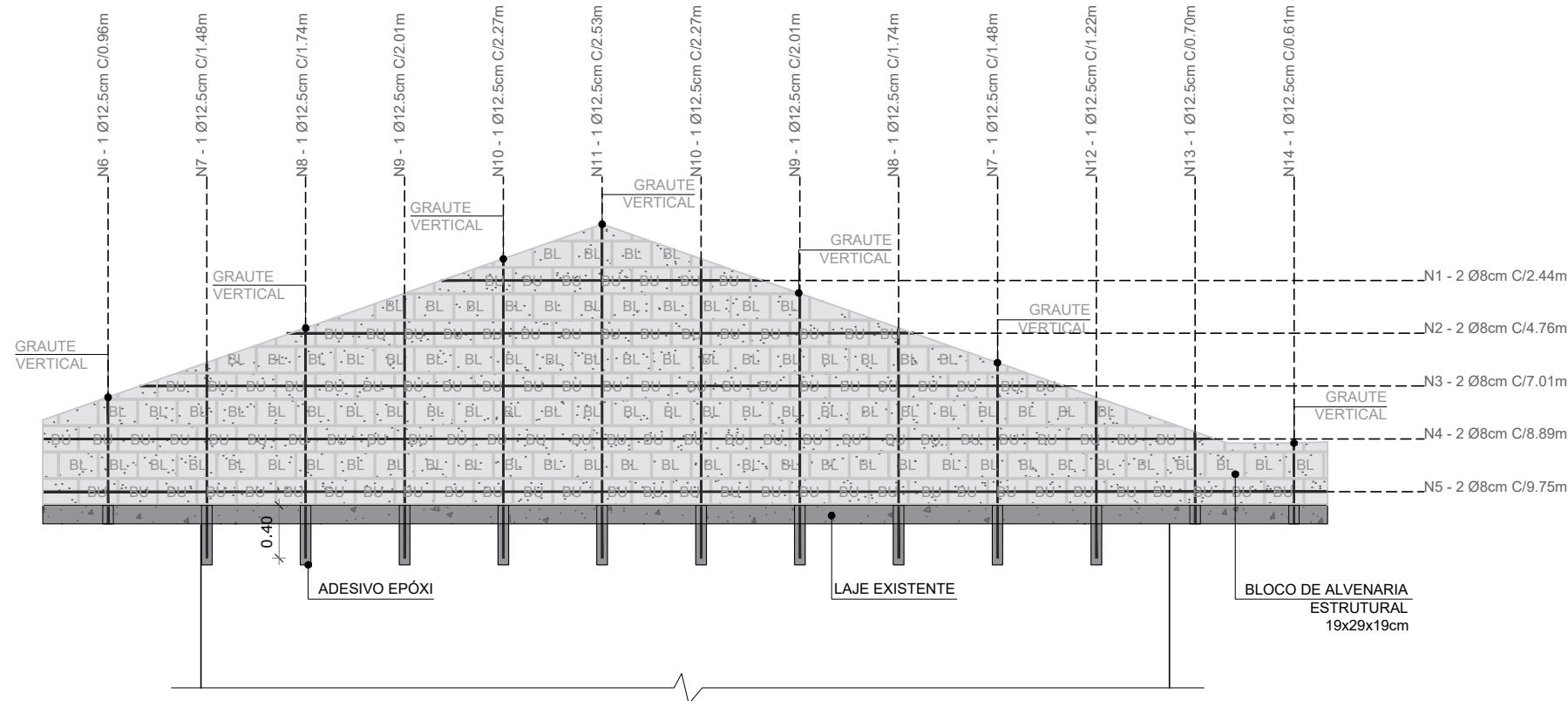
3 DETALHE 3 - OITÃO EM ALVENARIA ESTRUTURAL ESCALA 1/50
