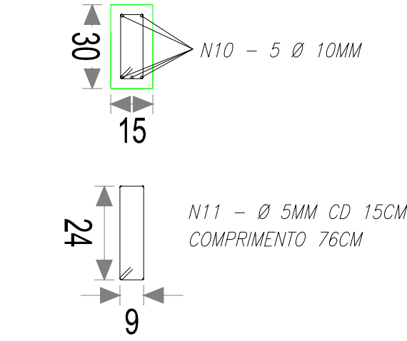
VIGA ESC. 1:20
