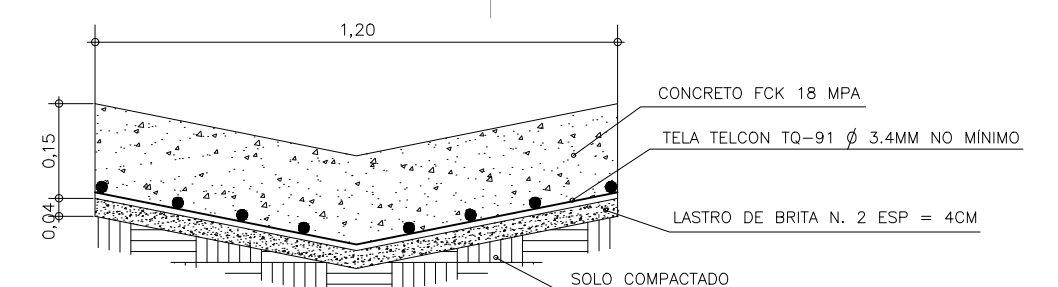
SARJETÃO EM CONCRETO ARMADO
