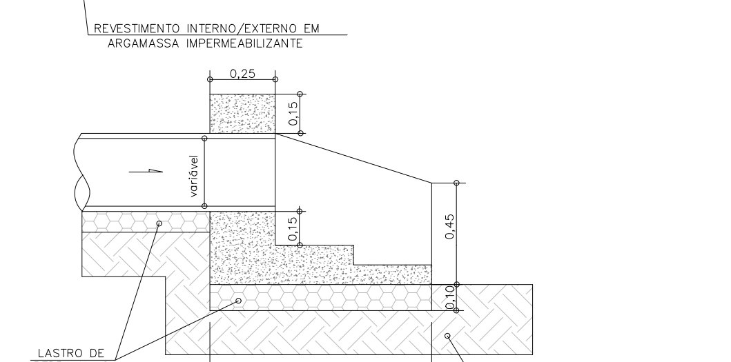
CORTE AA
