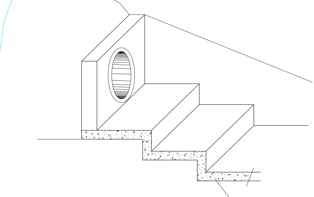
BOCA DE LOBO DUPLA
