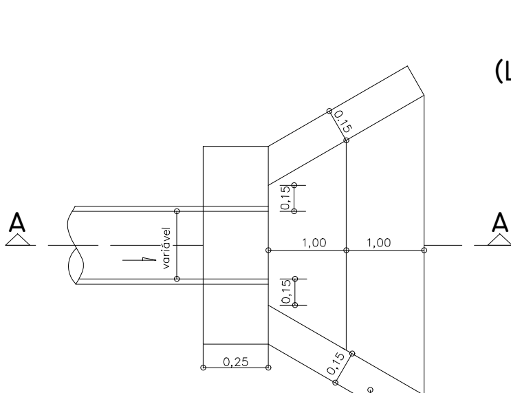
PLANTA
