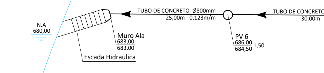
ESCALADA HIDRÁULICA - TIPO
