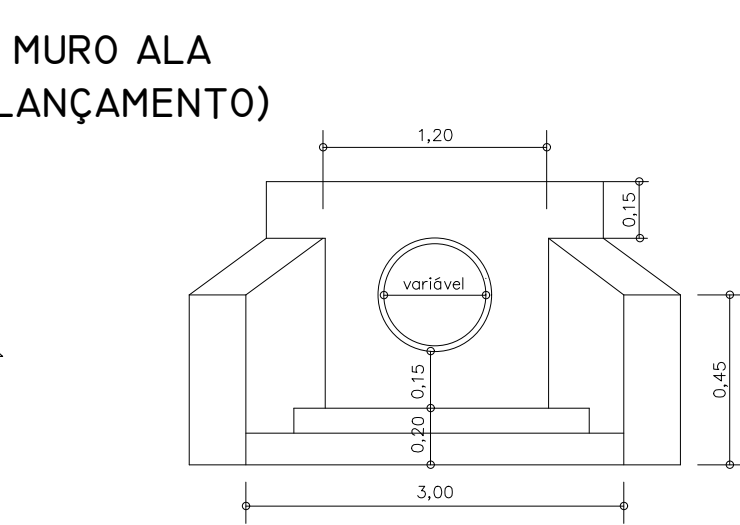
ELEVÇÃO
